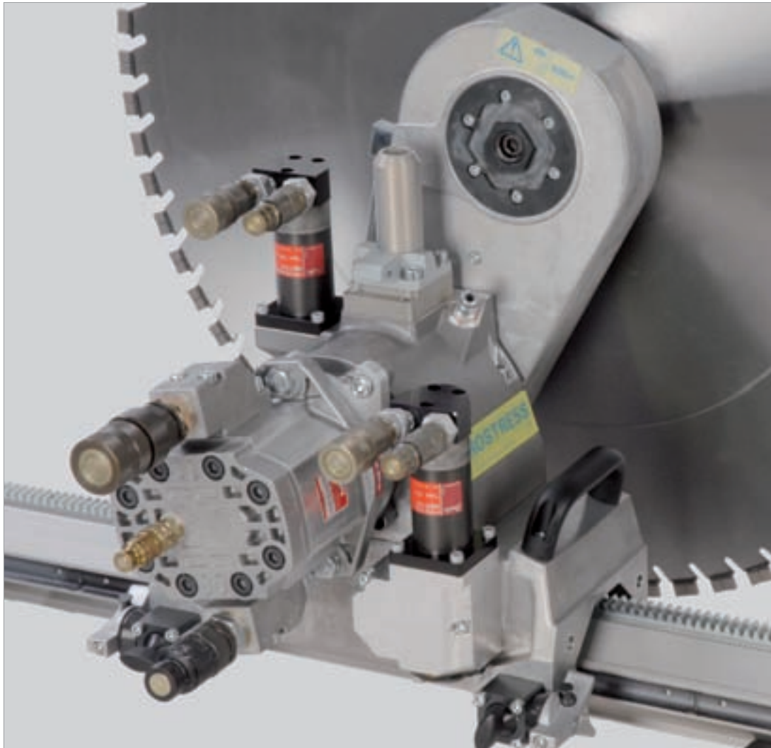
Kompakter Sägekopf mit Riemenschwenkarm
