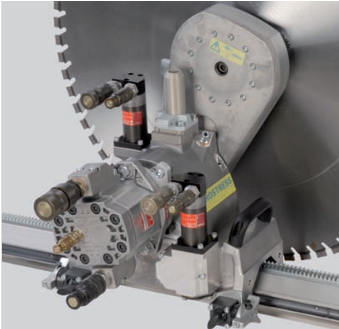
Hauptmotor mit Leckölanschluss
